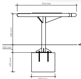
Fondation démontable
